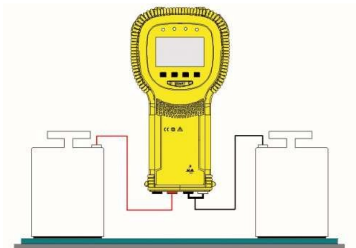
1. Pont-pont közti ellenállás mérése
