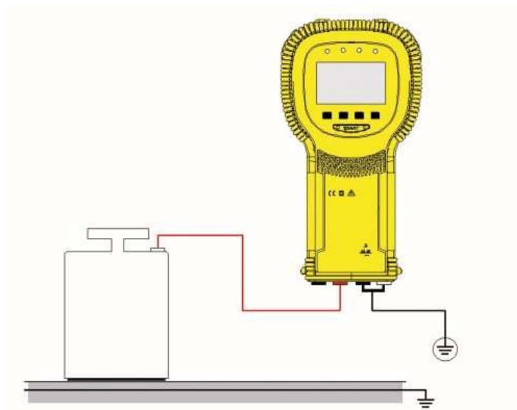
2. Földelési pontig mért ellenállás
